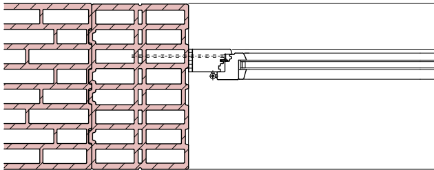
1re couche, demi-brique non coupée dans la zone de l'embrasure de fenêtre
