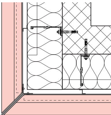
Profilé Quetschbug
