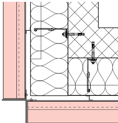
Profilé Kreuzeck
